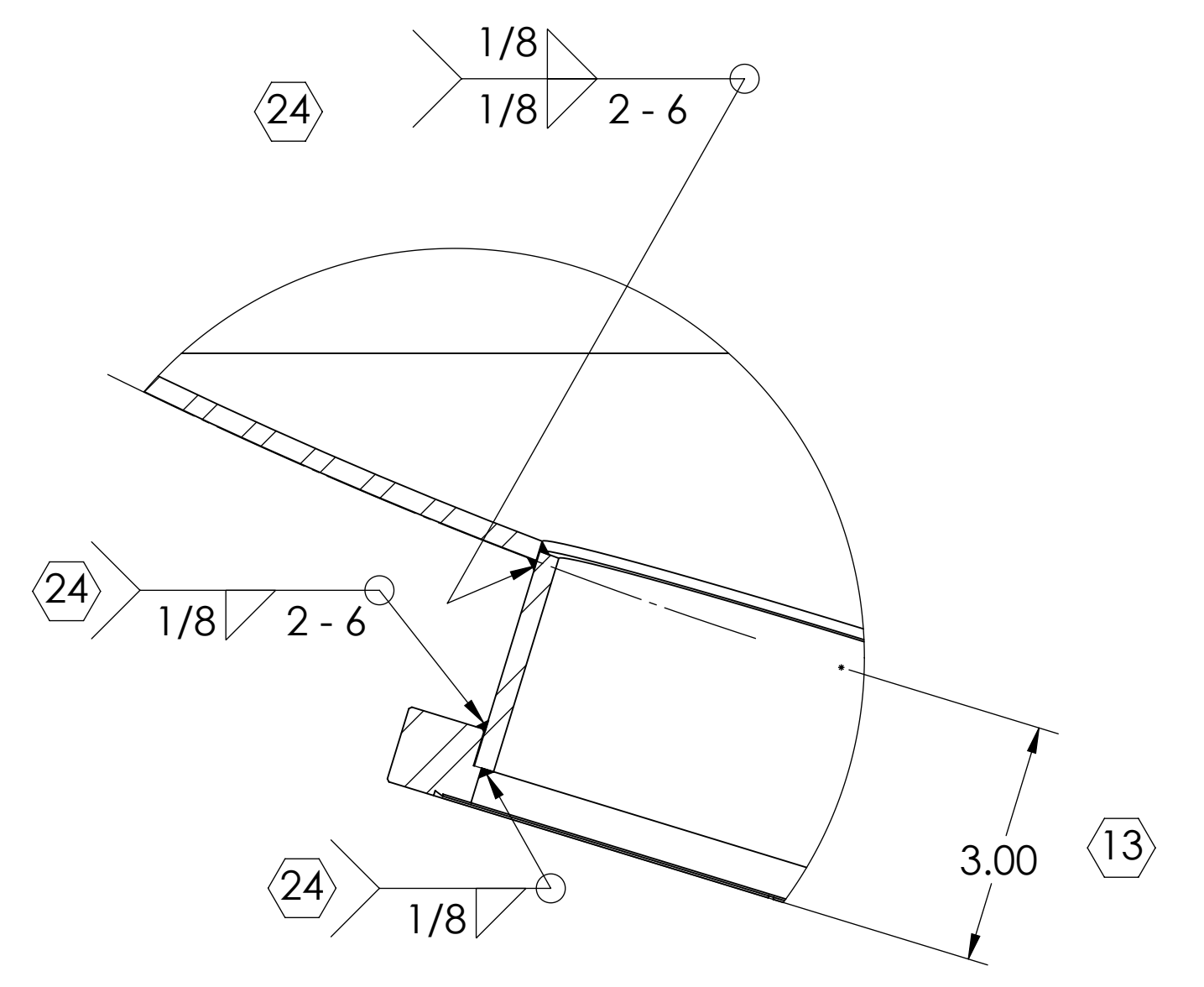
DETAIL D SCALE 1 : 2 3 PL.
