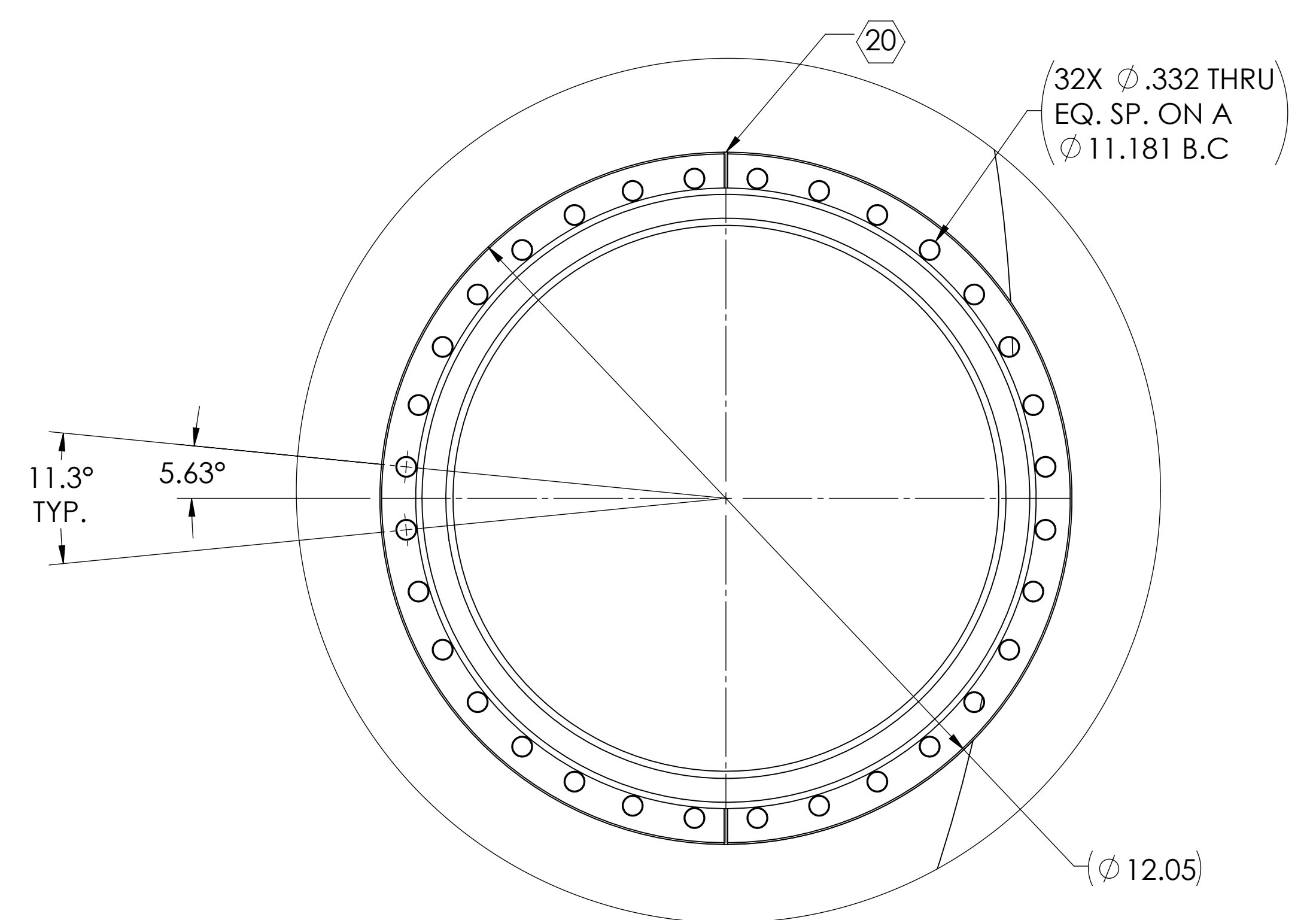
DETAIL E SCALE 1 : 2 2 PL.
