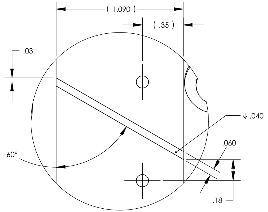
DETAIL C SCALE 2 : 1 2 PLCS
