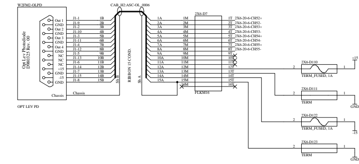
WA2K FM2 Opt Lever PD
