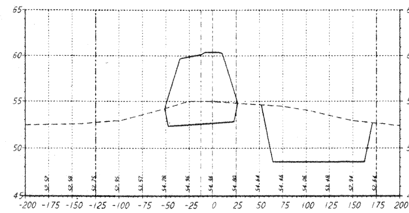
STA 70+00.00
