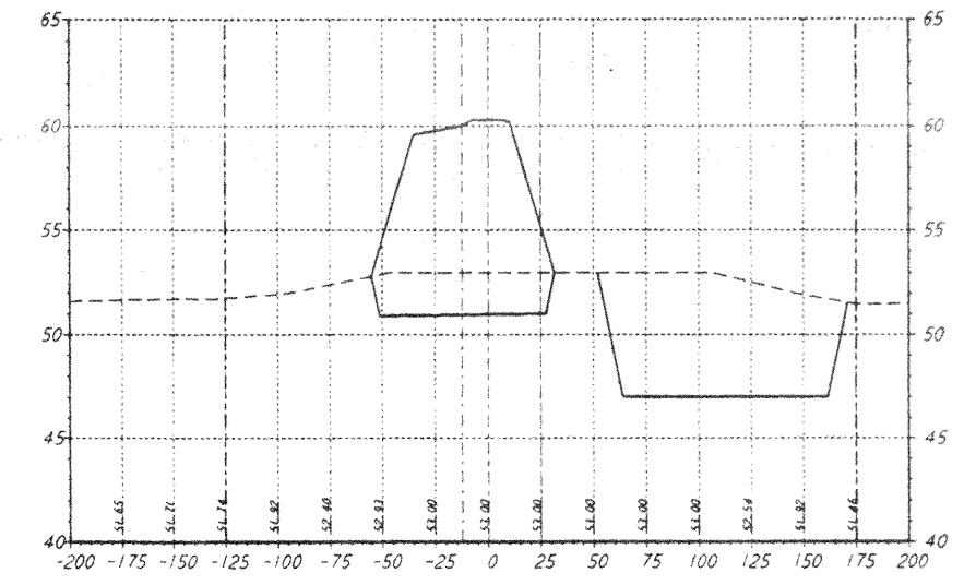
STA 74+00.00
