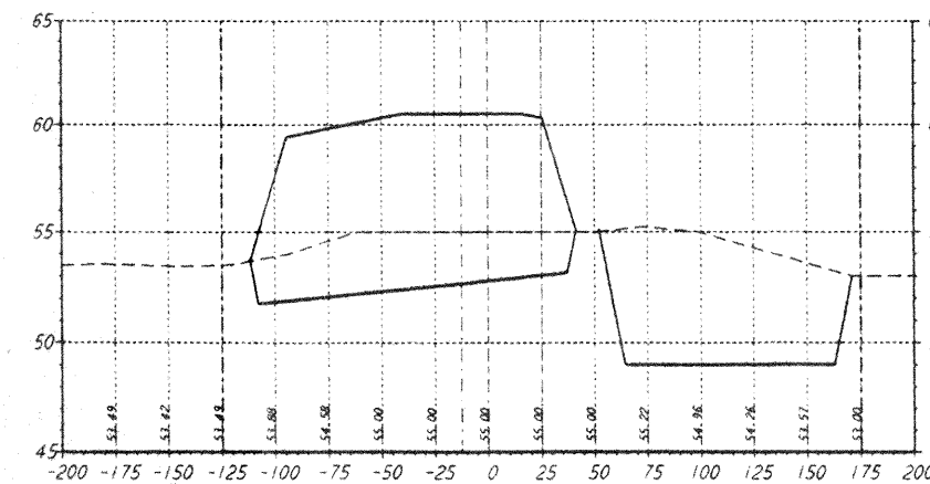
STA 66+00.00
