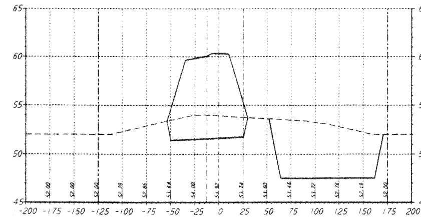
STA 72+00.00
