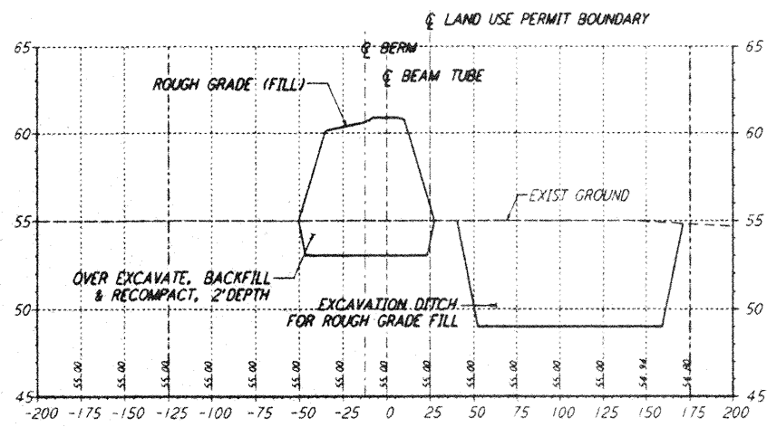
STA 56+00.00
