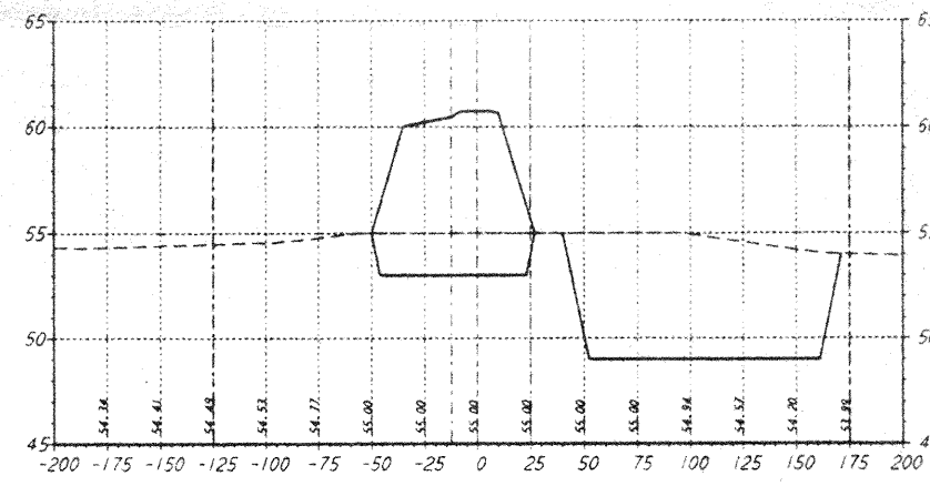
STA 60+00.00
