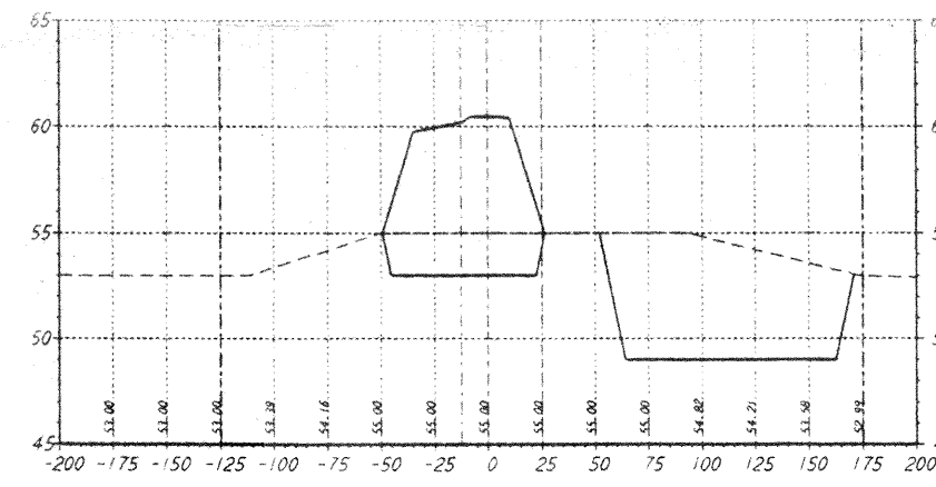
STA 68+00.00
