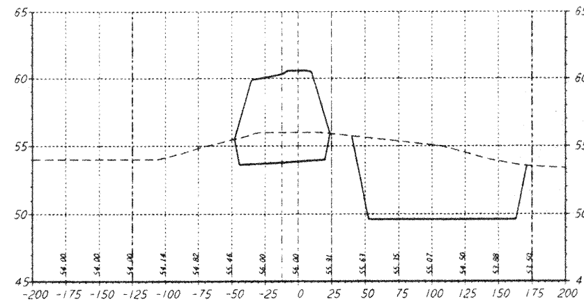
STA 64+00.00
