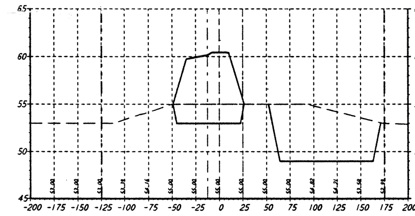
STA 68+00.00
