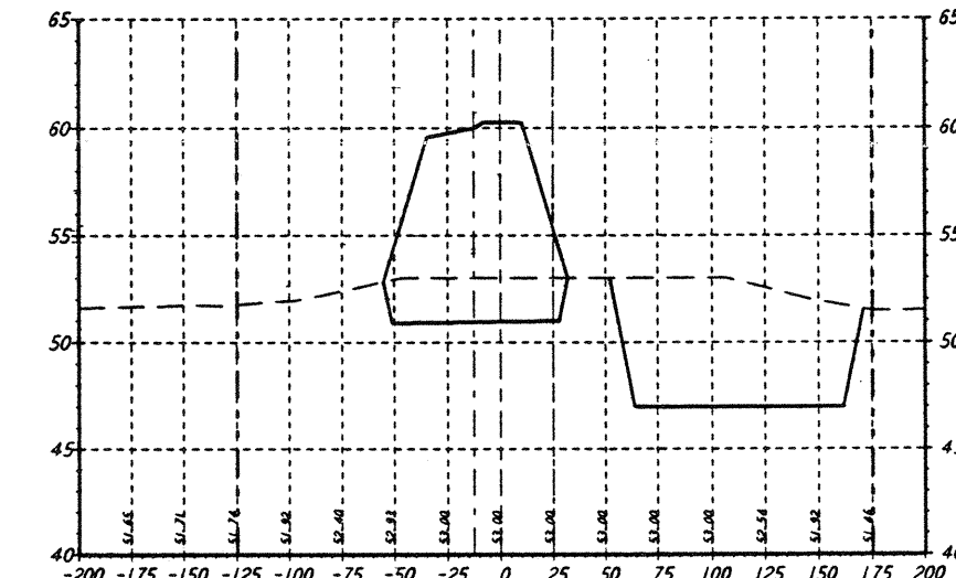
STA 74+00.00
