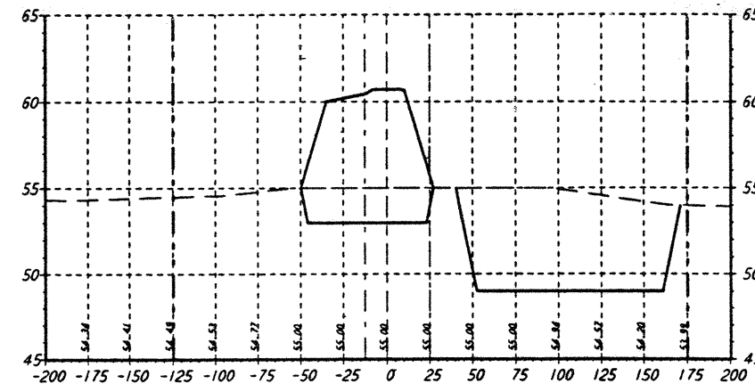
STA 60+00.00
