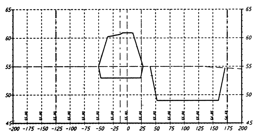
STA 54+00.00
