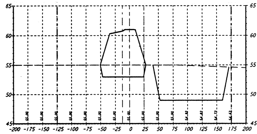
STA 52+00.00
