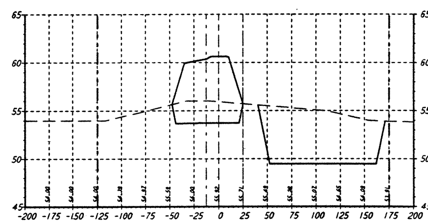
STA 62+00.00
