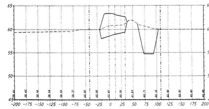
STA 124+00.00
