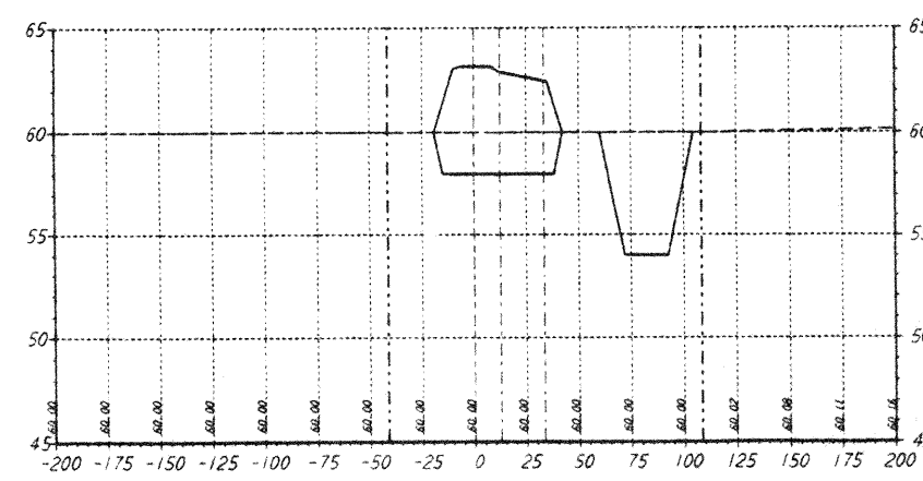
STA 116+00.00
