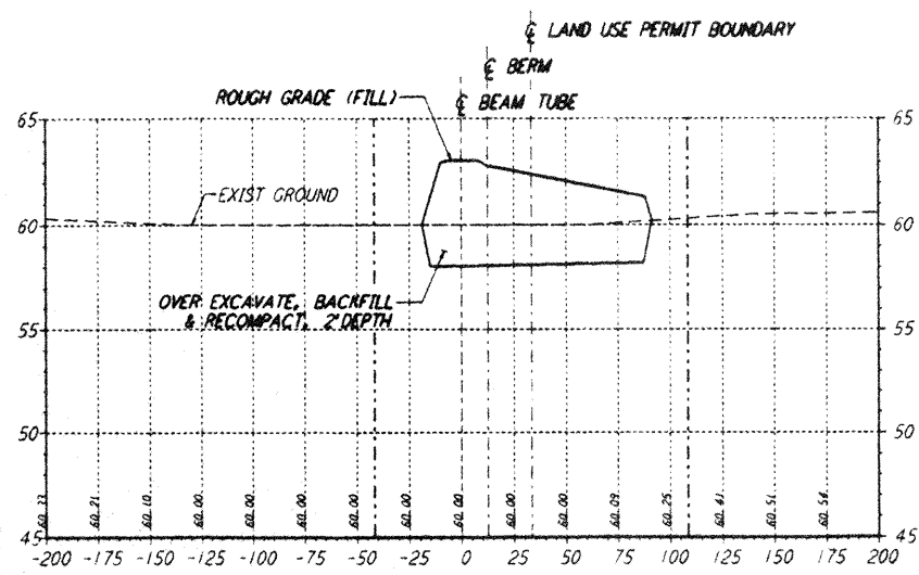
STA 114+00.00
