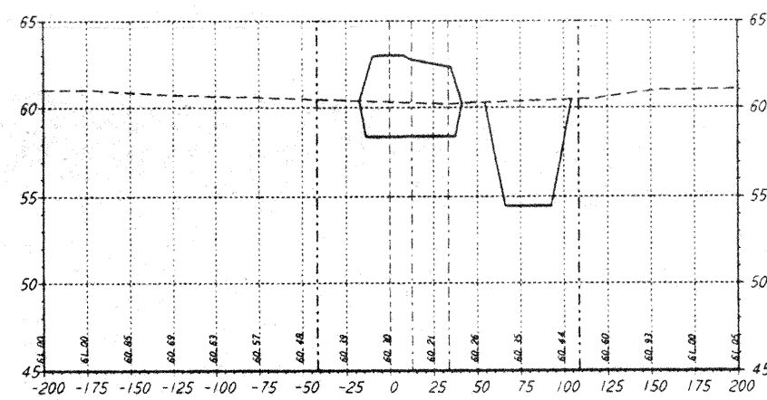
STA 110+00.00
