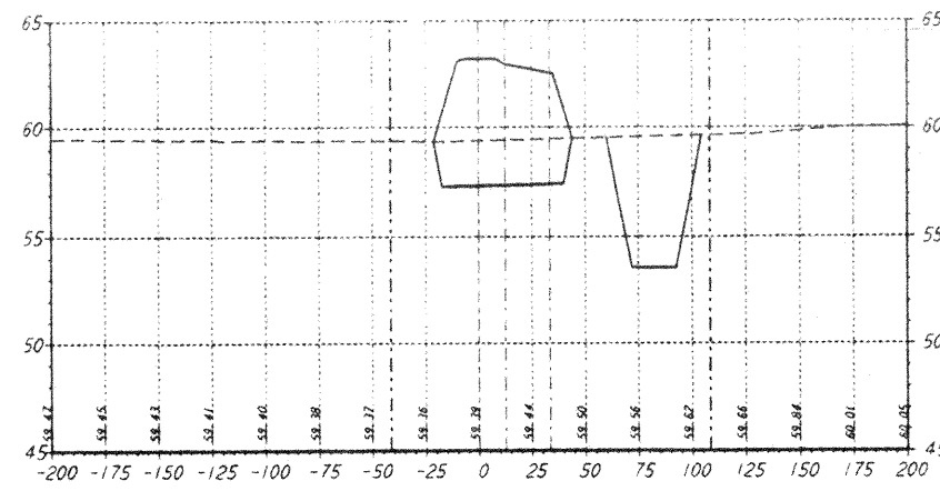
STA 118+00.00
