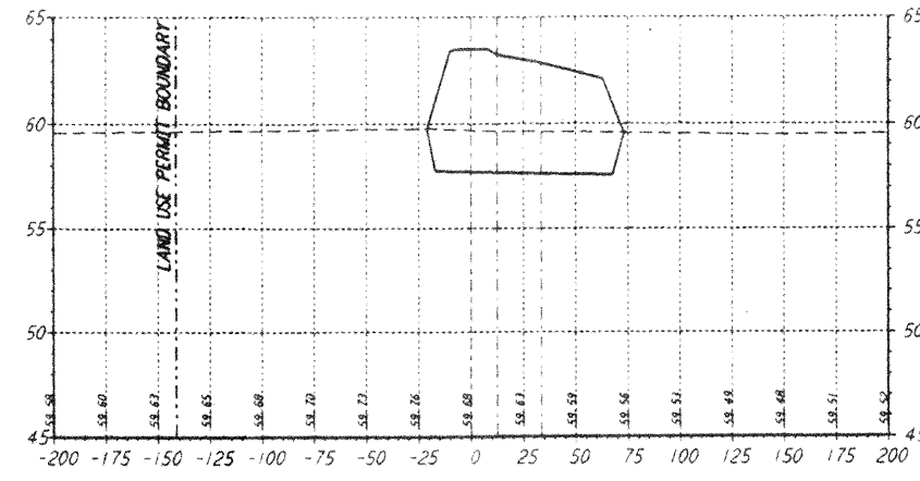
STA 130+00.00
