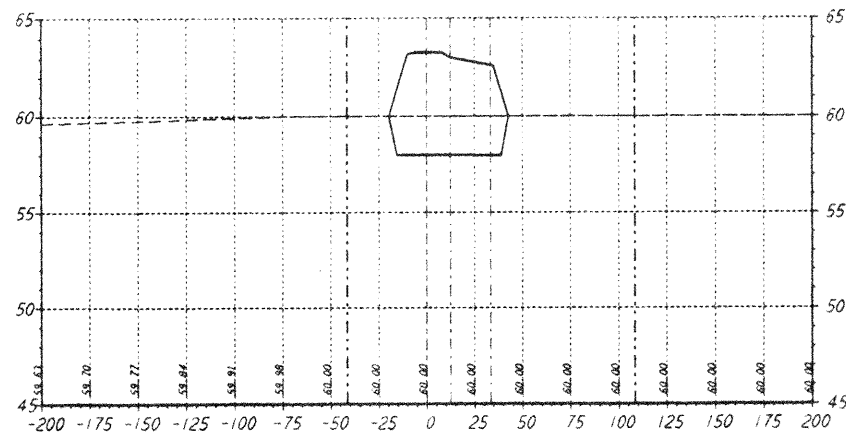
STA 122+00.00
