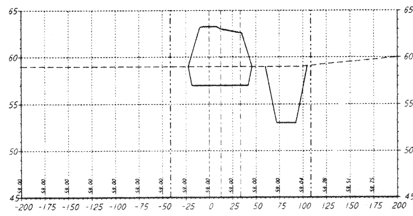
STA 120+00.00
