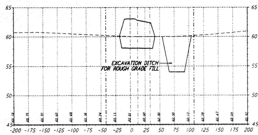
STA 112+00.00
