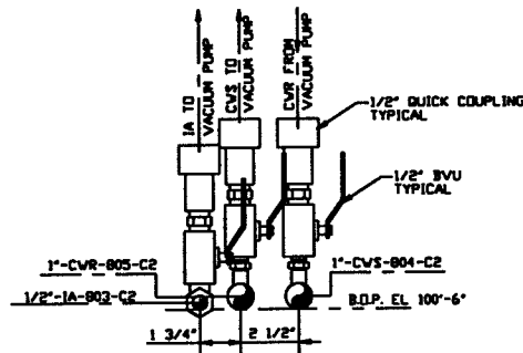
DETAIL 1 SCALE: 3"=1'-0" V049-5-021, SHT1
