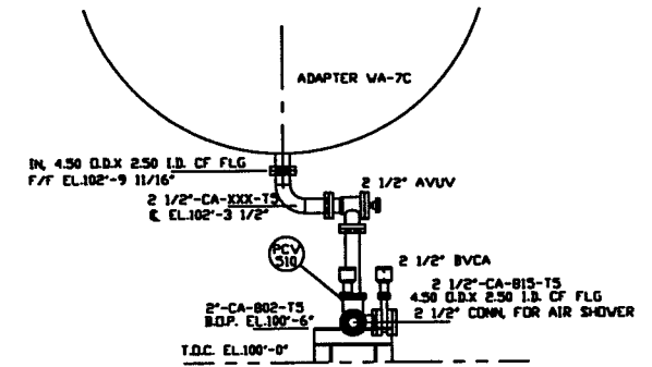
SECTION E SCALE: 3/4"=1'-0" V049-5-021, SHT1
