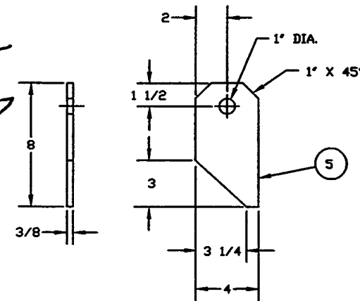
DETAIL "16" QTY: 4
