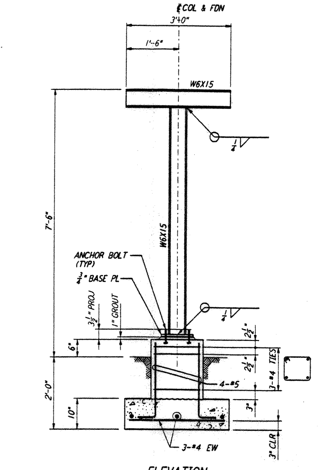
ELEVATION
