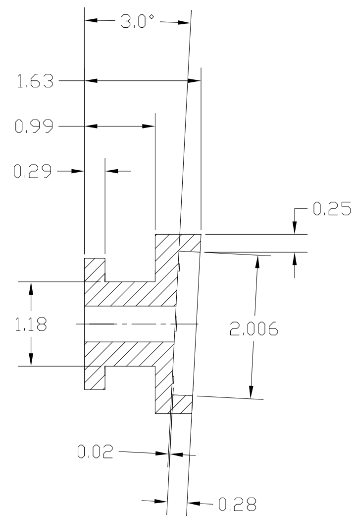
SECTION A-A
