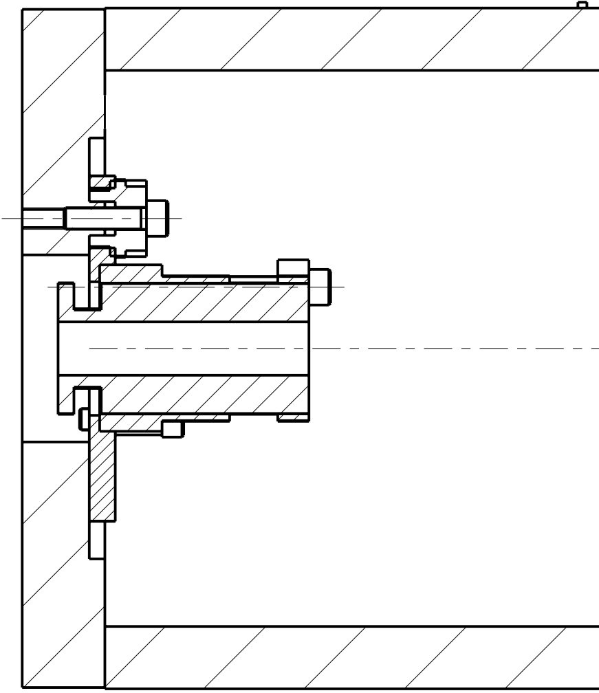
SECTION A-A
